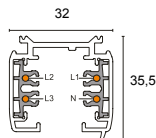
CARRIL TRIFÁSICO SUPERFICIE DE 2 METROS NEGRO CÓDIGO: 62504 BLANCO CÓDIGO: 62506 PVP: 59,95€
