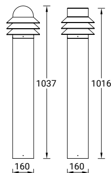
(1) Cúpula redondeada (2) Cúpula plana
