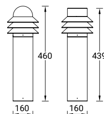
(1) Cúpula redondeada (2) Cúpula plana
