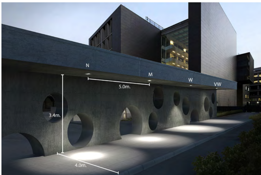
TAKEO 1 70780-W30 Beam: N/M/W/VW
