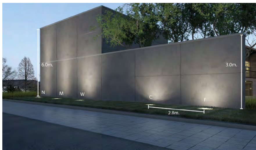
HARPER 1, 70031-W30 Ángulo: N/M/W (Setback 0.5m)
