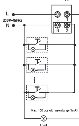
Diagrama de cableado conexión a 3 hilos
