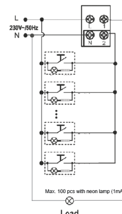
Diagrama de cableado conexión a 4 hilos
